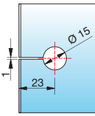
Bohrlochmaß bei 100°
