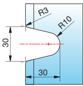
Randausschnitt R30
