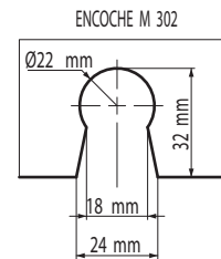
Encoche M302 pour pièce de fixation 3265 Partition clip notch
