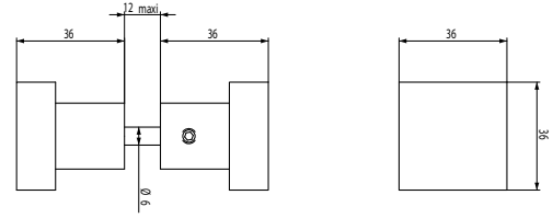
Pièce de fixation 3265.XX.05Q Partition clip for fixed panel
